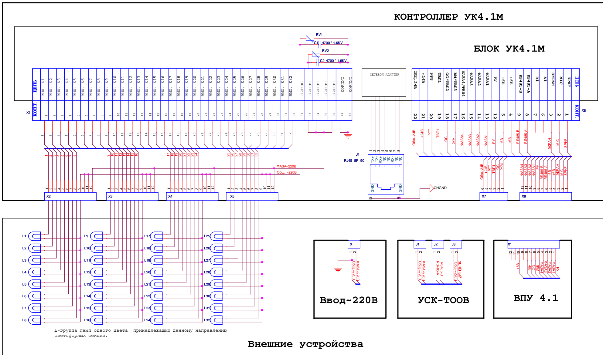
Рис. 2. Схема электрическая содинения УК4.1М со светофорными секциями, с УСК-ТООВ (Указателями Скорости или Табло Обратного Отчёта Времени) и с ВПУ4.1(Выносным Пультom диспетчерского Управления).
